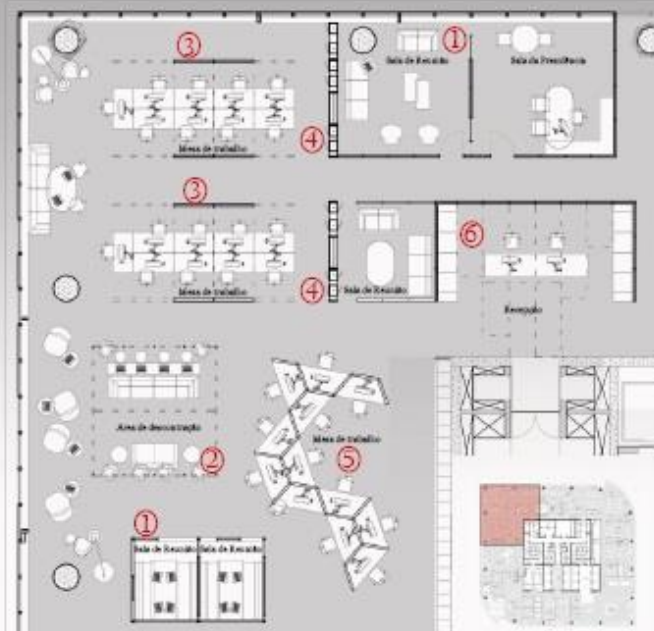
PLANTA DO SETOR AMPLIADA
